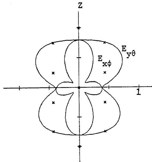
(d) three port voltages, compare with Fig. 13c.
